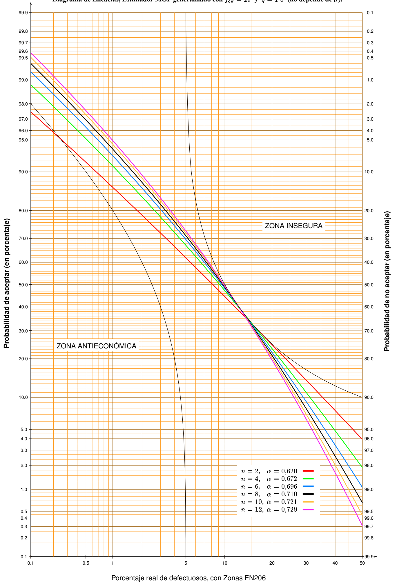
Diagrama de Eficacias, Estimador MOP generalizado con f_{ck} = 25 y q = 1,0 (no depende de \sigma ).
